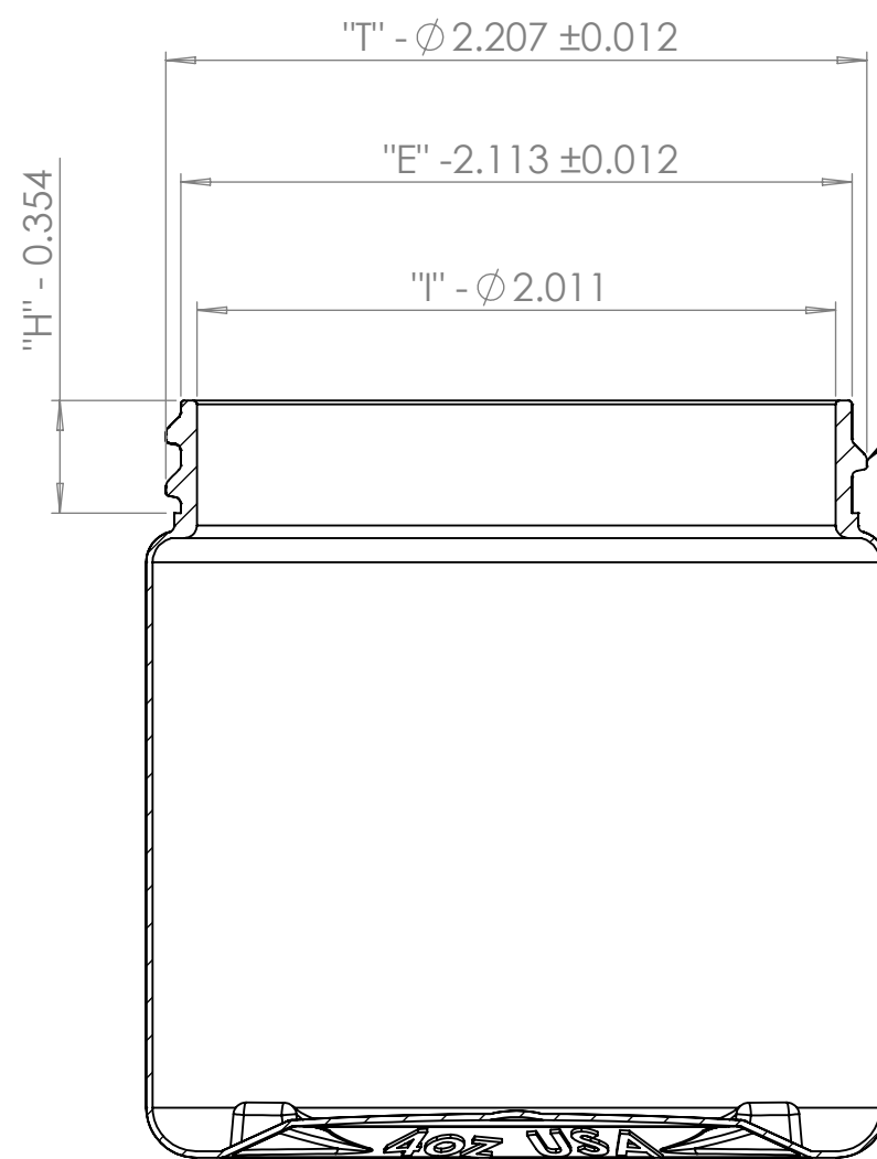
SECTION A-A
